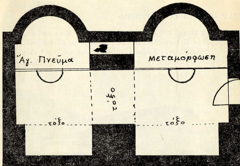
Εἰκ. 2. Πρόχειρο σχεδιάγραμμα κάτοψης τοῦ ναοῦ τοῦ Ἁγ. Πνεύματος.
